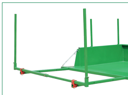
Ladeflächenverlängerung
